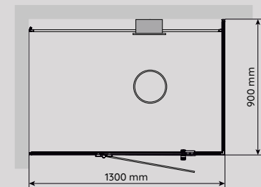
VISTA 130 HÖGER Mått: D 900 x B 1 300 mm
