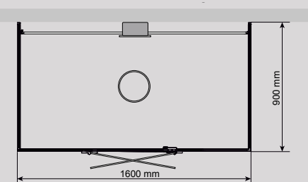
VISTA DCO 160 (VÄNSTER & HÖGER) Mått: D 900 x B 1 600 mm
