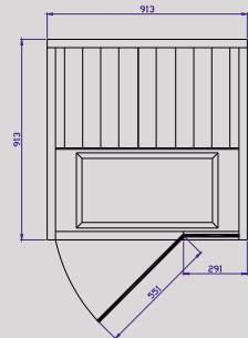
TYLÖSAND T-810 Mått: D 913 x B 913 mm Effekt: 1350 W
