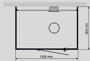
VISTA DCO 130 HÖGER Mått: D 900 x B 1 300 mm
