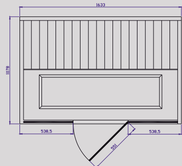
TYLÖSAND T-825 Mått: D 1 078 x W 1 633 Effekt: 1980 W
