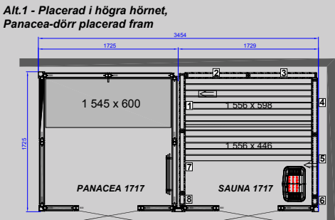
TWIN PANACEA 1717 Mått: D 1 725 x B 3 454 mm
