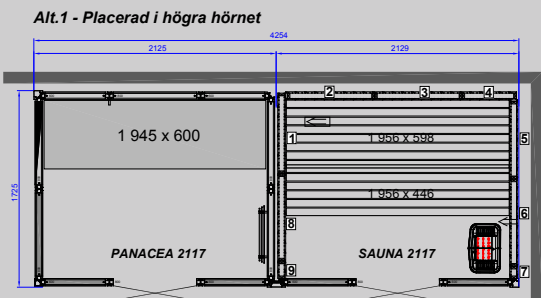
TWIN PANACEA 2117 Mått: D 1 725 x B 4 254 mm
