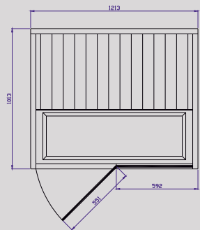
TYLÖSAND T-820 Mått: D 1 013 x B 1 213 mm Effekt: 1470 W
