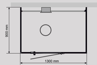
VISTA DCO 130 VÄNSTER Mått: D 900 x B 1 300 mm
