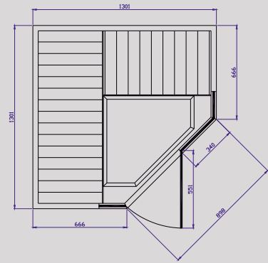
TYLÖSAND T-870 Mått: D 1 301 x B 1 301 mm Effekt: 1600 W
