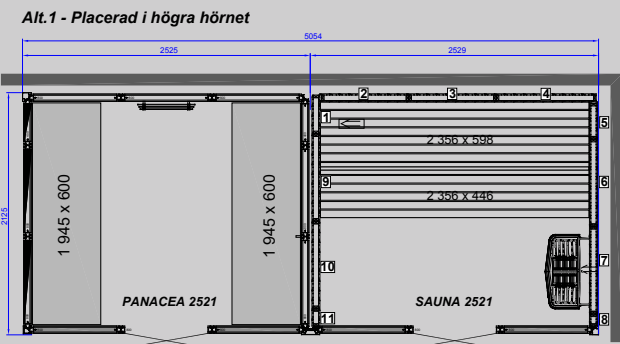
TWIN PANACEA 2521 Mått: D 2 125 x B 5 054 mm
