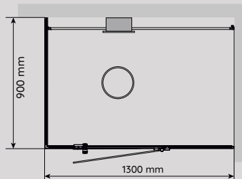
VISTA 130 VÄNSTER Mått: D 900 x B 1 300 mm
