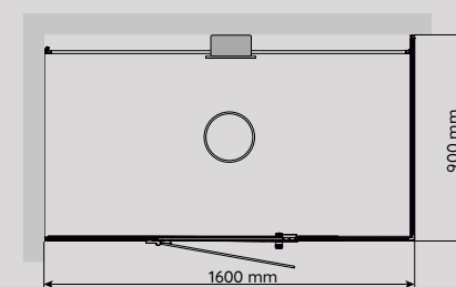
VISTA 160 HÖGER Mått: D 900 x B 1 600 mm
