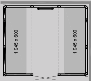
PANACEA 2521 2B Mått: 2 525 x 2 125 x 2 090 mm
