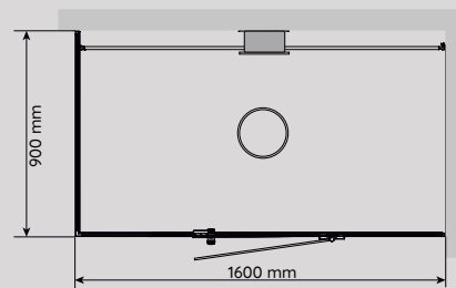
VISTA 160 VÄNSTER Mått: D 900 x B 1 600 mm
