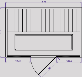
TYLÖSAND T-825 Size: D 1 078 x W 1 632 mm Power: 1980 W
