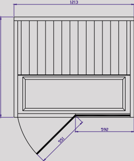
TYLÖSAND T-820 Size: D 1 013 x W 1 213 mm Power: 1470 W
