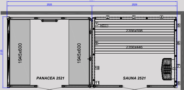
TWIN PANACEA 2521 Maße: T 2125 x B 5054 mm
