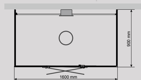
VISTA DCO 160 (LINKS & RECHTS) Maße: T 900 x B 1600 mm
