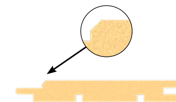
1. SAUNA-WANDVERKLEIDUNG MIT STP-PROFIL
