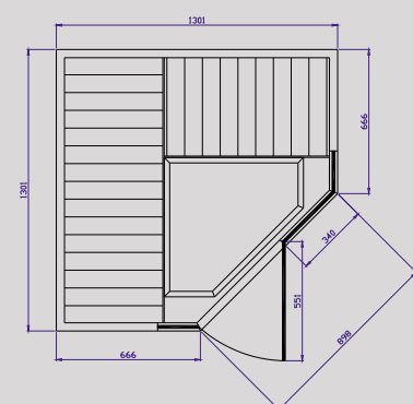
TYLÖSAND T-870 Maße: T 1301 x B 1301 mm
