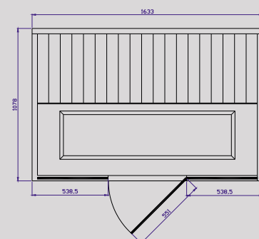
TYLÖSAND T-825 Maße: T 1078 x B 1633
