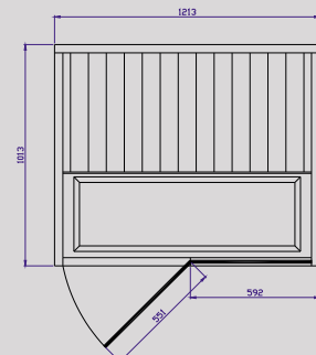
TYLÖSAND T-820 Maße: T 1013 x B 1213 mm
