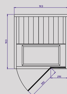
TYLÖSAND T-810 Maße: T 913 x B 913 mm
